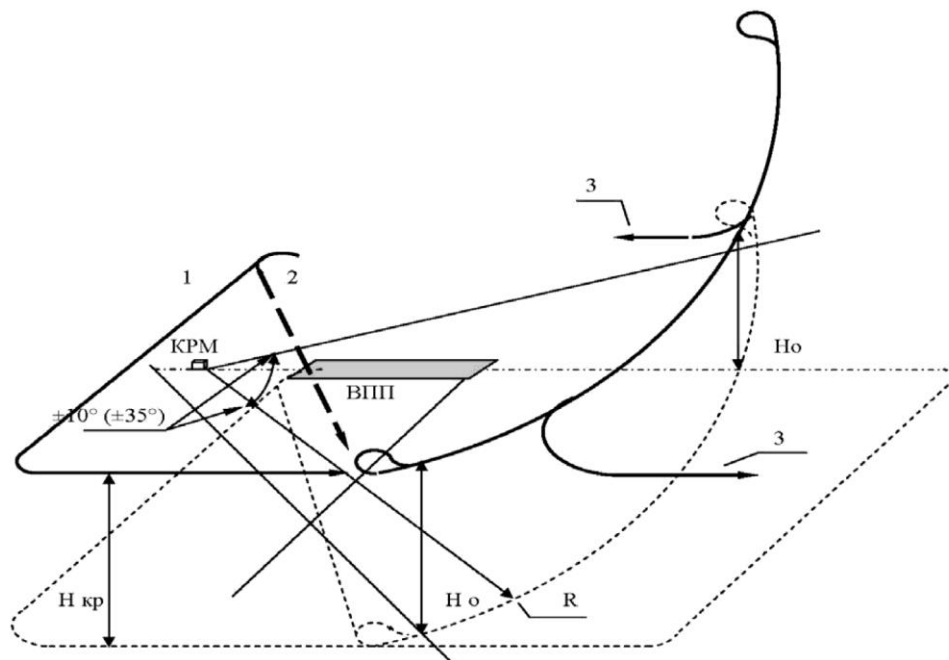
Рис. 1.2. Траектория полета при определении 3Д КРМ в горизонтальной плоскости и напряженности поля в 3Д КРМ под углами \pm 10^\circ (\pm 35^\circ)
