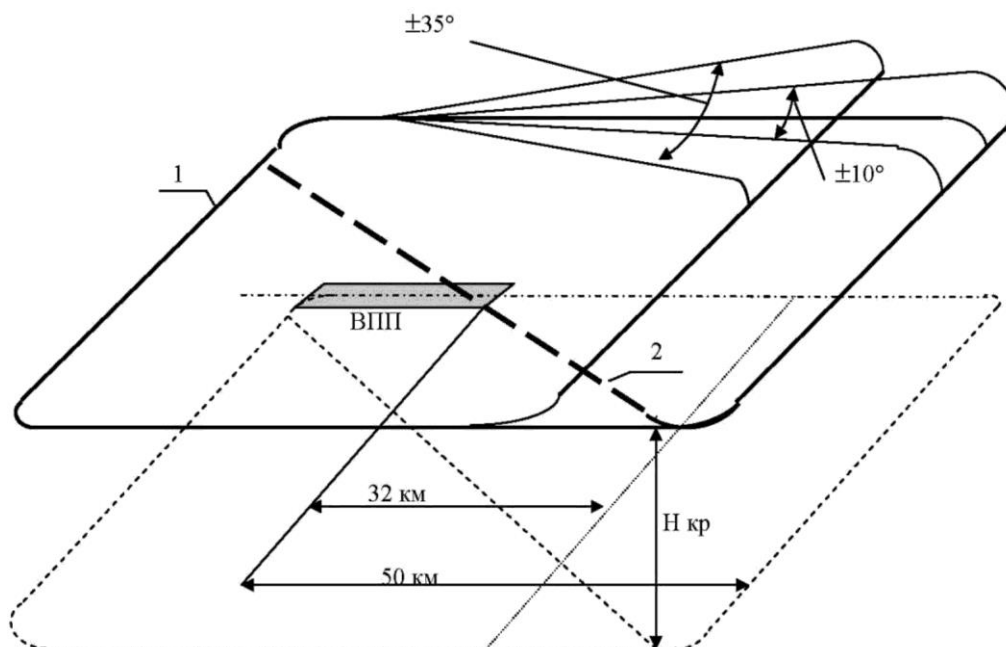
Рис. 1.4. Траектория полета при определении ЗД КРМ в вертикальной плоскости 1 – траектория захода по установленной схеме; 2 – траектория по согласованию с органом ОВД; H кр – установленная высота полета по схеме или безопасная высота.
