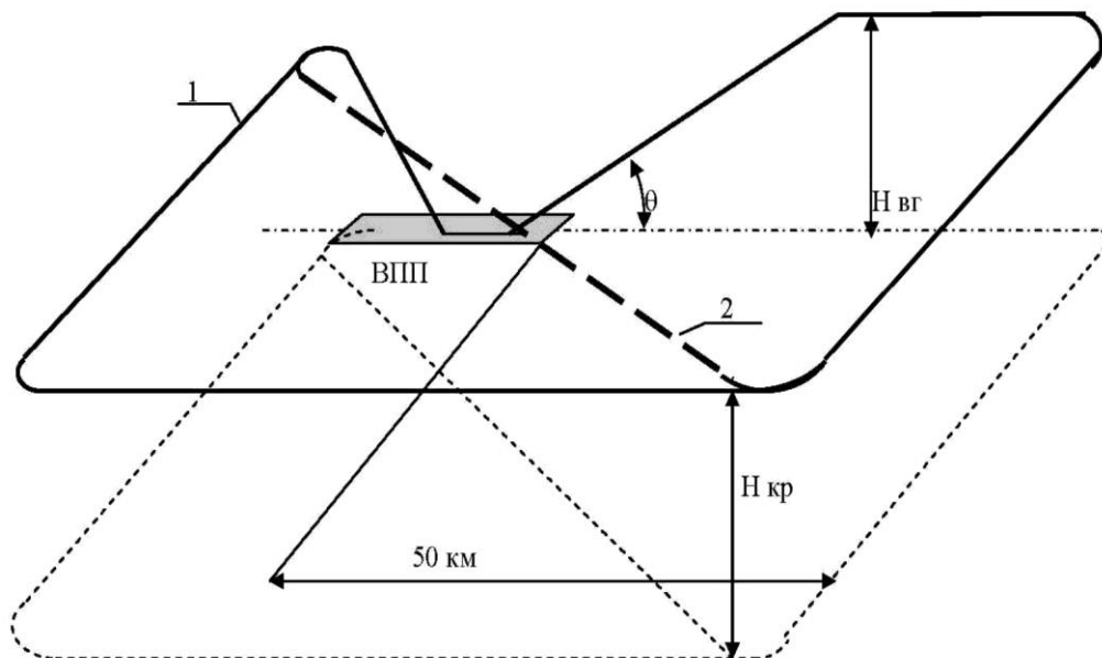
Рис. 1.3. Траектория полета при определении ЗД КРМ в горизонтальной (вертикальной) плоскости под углом 0^\circ относительно осевой линии ВПП.
