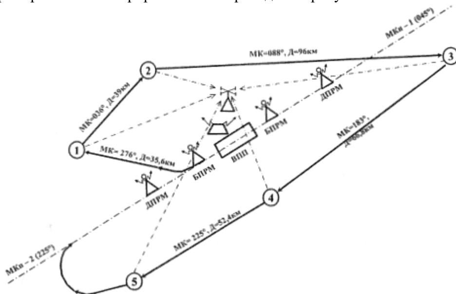
18.5. Пример схемы маневрирования ВС при полете над контрольными ориентирами (геодезическими знаками).
